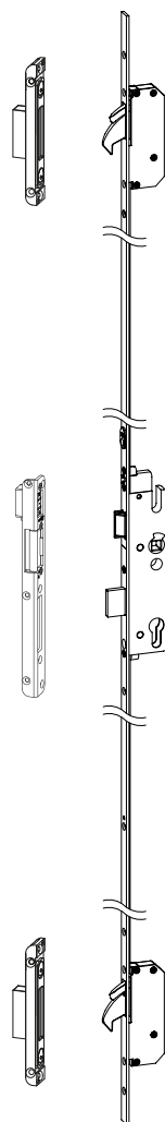
AV4D Automatik Verriegelung mit Tagesfallen Funktion 3 - fach mit 2 Haken , Farbe Topzink Tag / Nacht Funktion - für temporär flexibles Ein- und Austreten ohne Schlüsseldrehung
