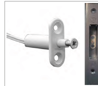
RIEGELSCHALTCONTACT Im Schliessblech eingebaut. Wird durch den Riegel im Schloss betätigt. Rückmeldung: Tür manuel oder mechanisch abgeschlossen!
