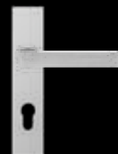
ELXQ PZ72 71 Schildmaße: 200x40x10 mm ED46 71
