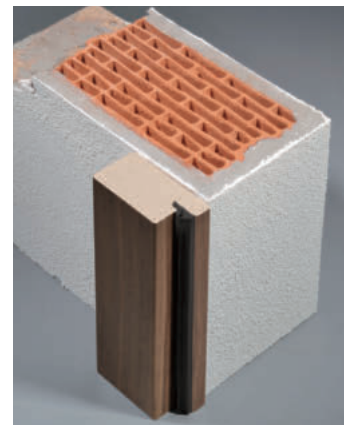
BLENDRAHMEN BM 45 auf der Wand, vor der Laibung montiert
