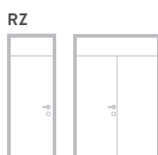
Raumhohe Zarge mit Querteil mit Kämpfer bis Stocklichthöhe von 2.520 mm (einflügelig, zweiflügelig)
