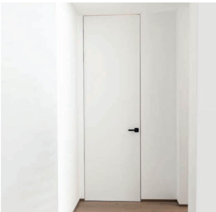
KONTEXT 46 in raumhoher Ausführung
