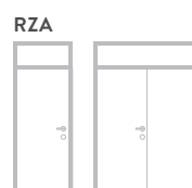
Raumhohe Zarge mit Querteil, Kämpfer und Oberlichte bis Stocklichthöhe von 2.520 mm (einflügelig, zweiflügelig)
