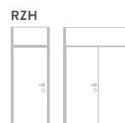
Raumhohe Zarge ohne Querteil mit Kämpfer und Oberlichte bis Raumlichte von 2.600 mm (einflügelig, zweiflügelig)
