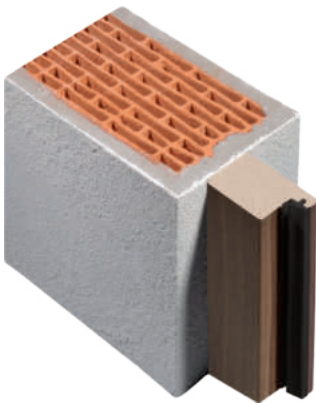
RAHMENSTOCK S-INTERIOR 46 in der Laibung montiert (beliebige Position)
