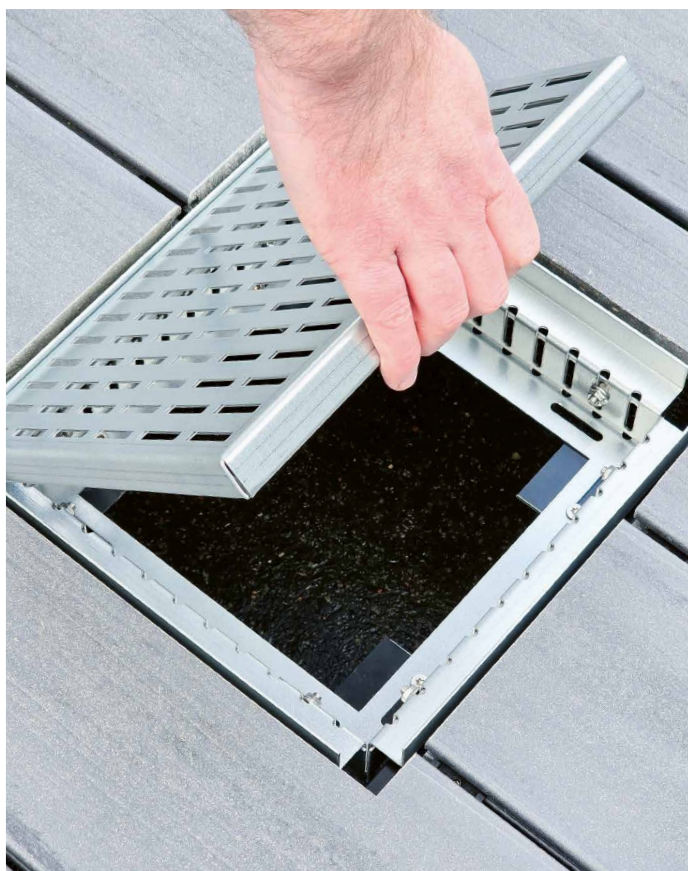
Abdeckblech in den montierten Kasten einlegen
