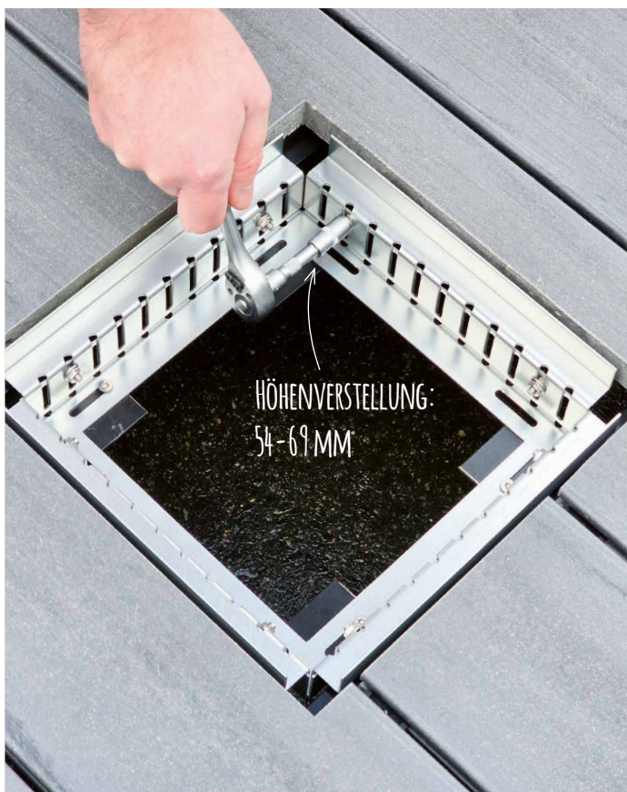
Höhe des Revisionskastens an den Terrassenbelag anpassen
