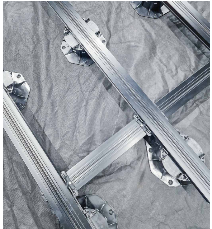
Konstruktion mit doppelter Unterkonstruktion am Anfang und Ende
